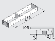
ORGA-LINE lokerikko, lev. 210 mm Harmaa/rst ZSI500FI1
