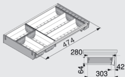
ORGA-LINE lokerikko, lev. 280 mm Harmaa/rst ZSI500BI3
