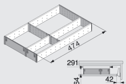
ORGA-LINE lokerikko, lev. 280 mm Harmaa/rst ZSI500FI3
