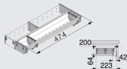
ORGA-LINE lokerikko, lev. 210 mm Harmaa/rst ZSI500KI2
